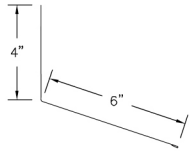
①① ABS Endwall (ABSEWcc)
