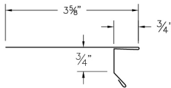
⑥① Drip Edge (ABSDEcc)
