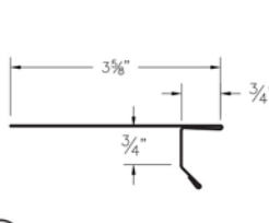
⑹ Drip Edge (DEcc)
