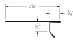
⑶ Drip Edge (DEcc)
