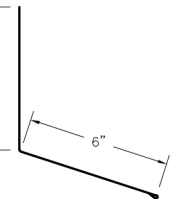
⑪ Universal Endwall (EWcc)
