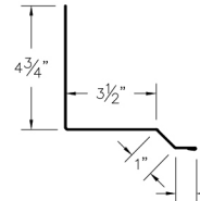
⑧ Universal Sidewall (SWcc)
